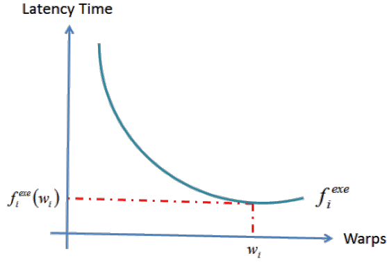
圖 8 不同 Warp 數所花的 Latency Time
