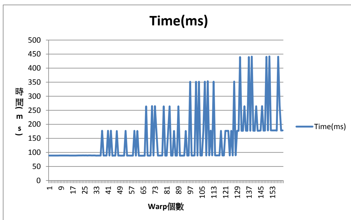
圖 7 Warp 個數與執行時間的關係
