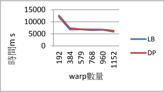
圖 9 Warp 數量與執行時間的關係
